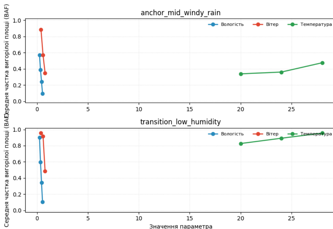
Рис. 4.2.1 – Криві однофакторної чутливості середньої частки вигорілої площі до зміни вологості, температури та сили вітру
