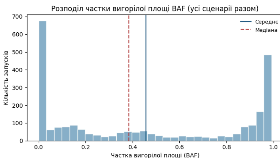
Рис. 4.4.1.1 – Розподіл частки вигорілої площі по всіх сценаріях серії глобальної чутливості
