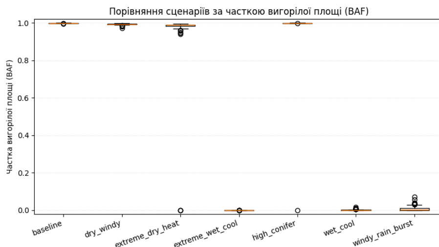
Рис. 4.1.2 – Порівняння сценаріїв за часткою вигорілої площі BAF (діаграми розмаху)
